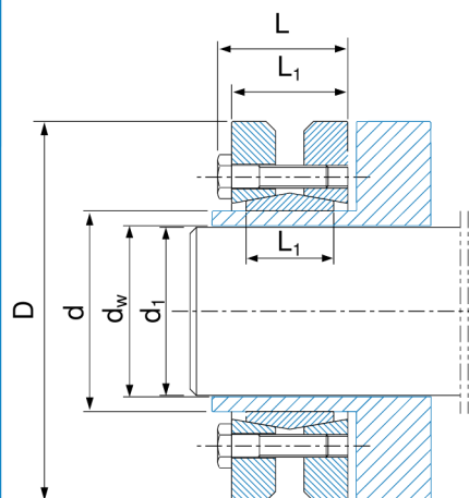
tuleja BK19
