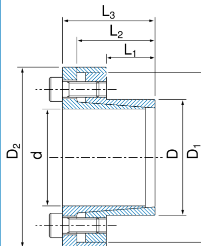
Tuleja mocująca BK80
