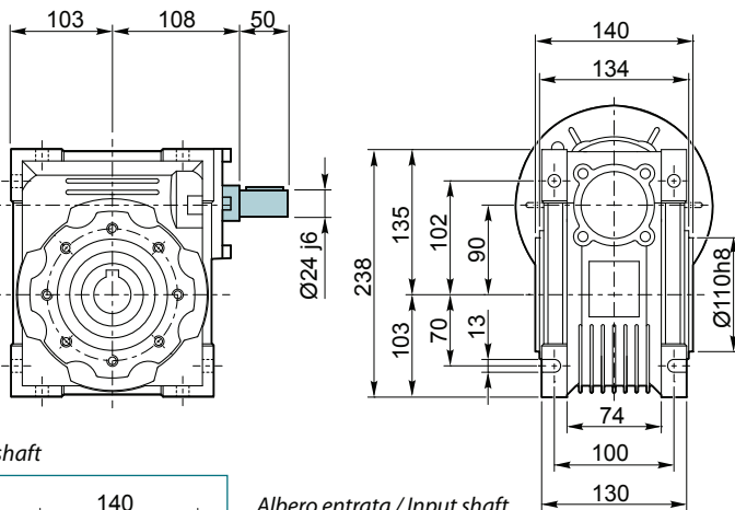
Albero entrata / Input shaft
